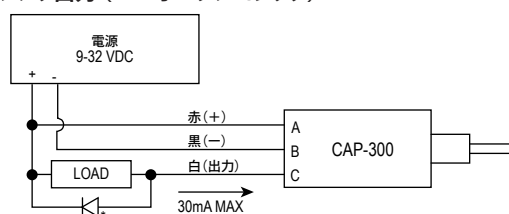
シンク出力 (NPNオープンコレクタ)
