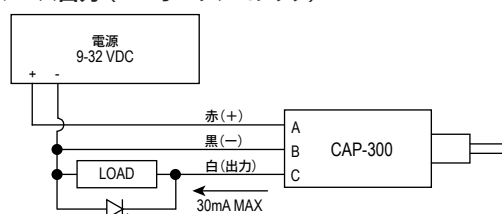
ソース出力 (PNPオープンコレクタ)
