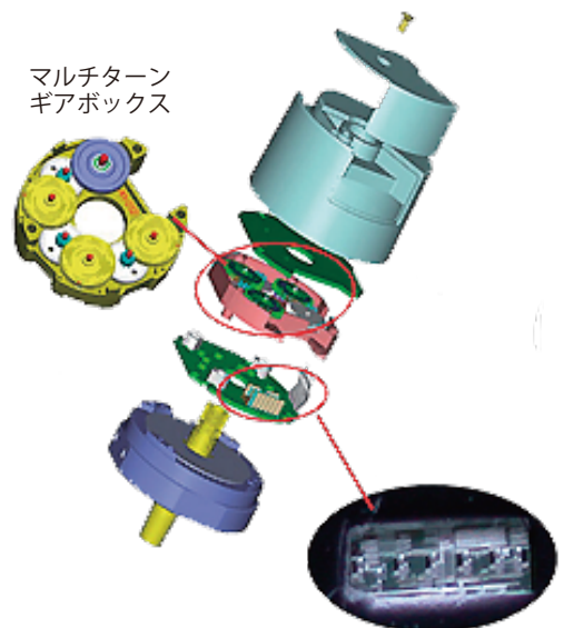
光学系一体型ASIC
