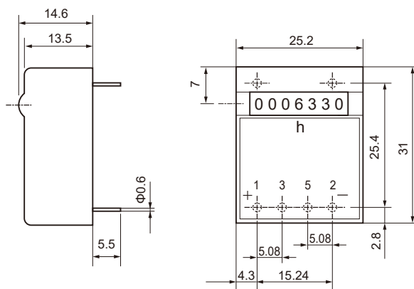
形状タイプ0 (基板実装)
