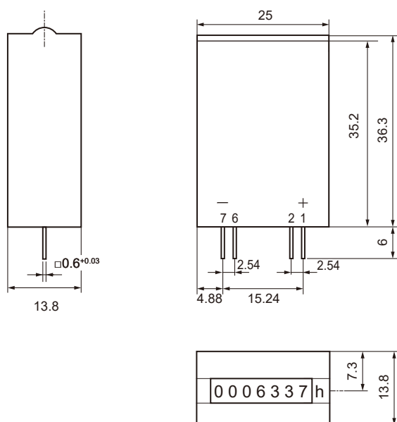
形状タイプ7 (プラグイン)
